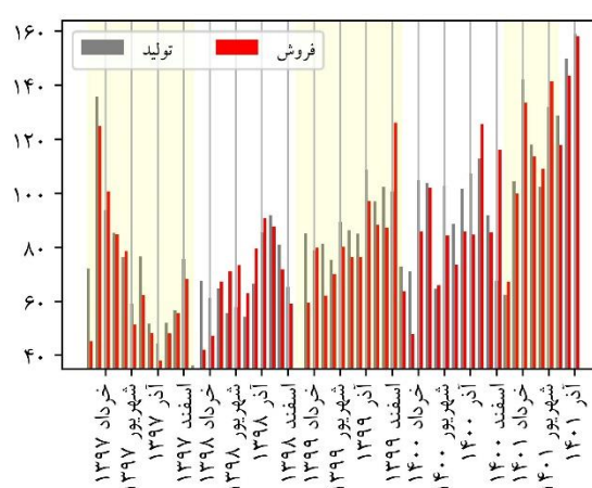
نمودار ۸. شاخص‌های تولید و فروش بخش خودرو و قطعات (۱۰۰=۱۳۹۵)
