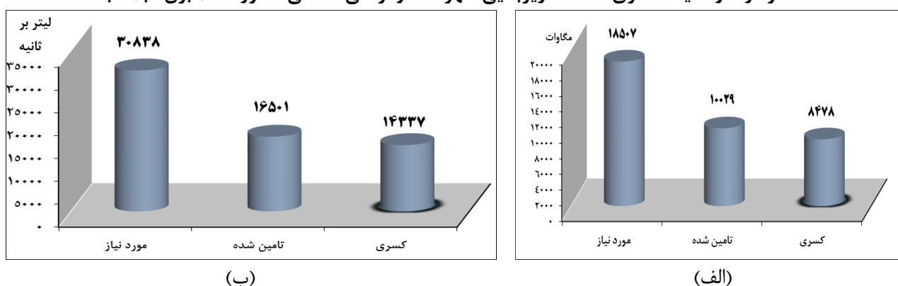
نمودار ۱. وضعیت کسری امکانات زیربنایی شهرک‌ها و نواحی صنعتی کشور؛ الف) برق، ب) آب
