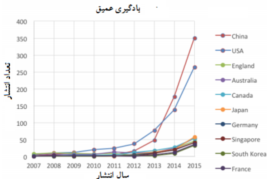
شکل ۱. مقالات مجلات علمی به تفکیک کشورها که در آنها عبارت‌های «شبکه عصبی» یا «یادگیری عمیق» ذکر شده
