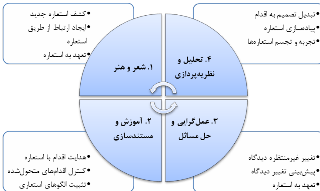
شکل ۲. چارچوب دوازده مرحله‌ای استفاده از استعاره‌ها در حکمرانی [۳۰]
